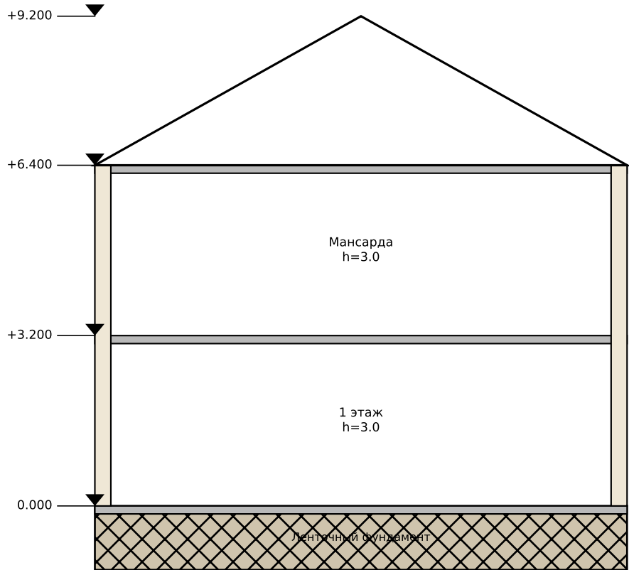
Разрез 1-1
