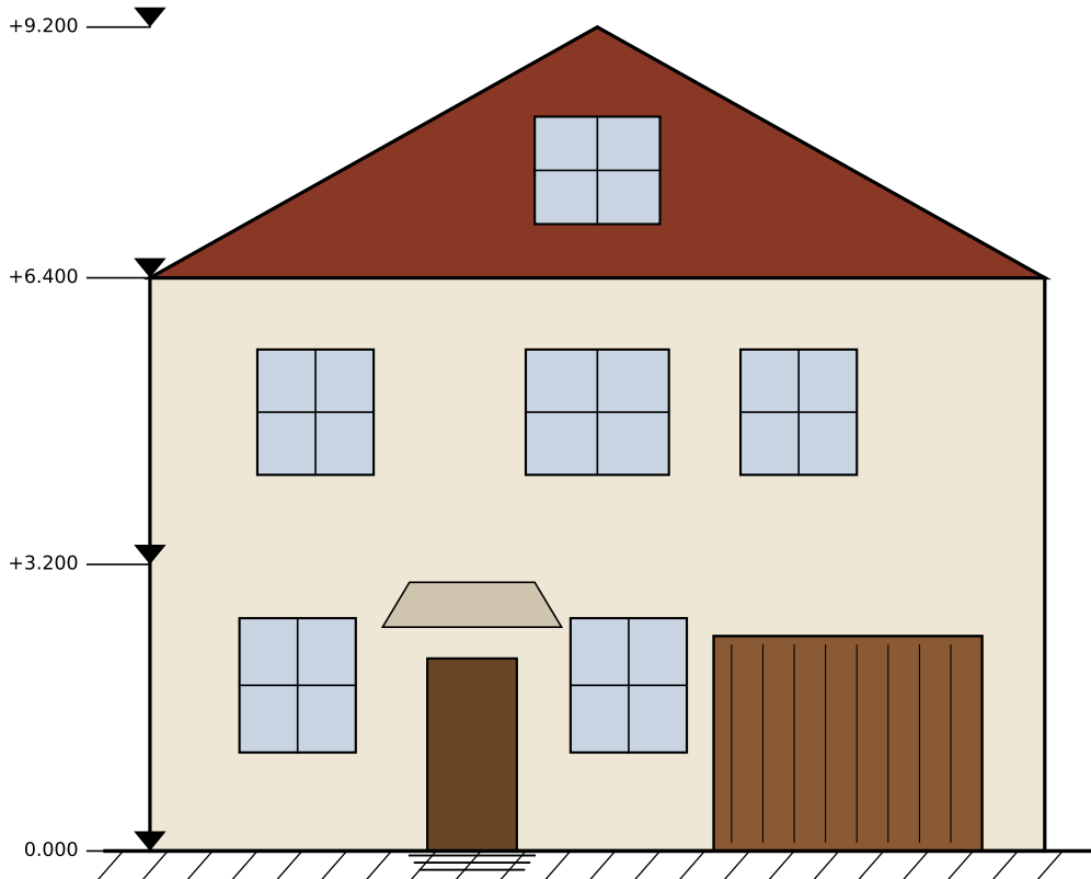
Фасад 1-7 (главный)
