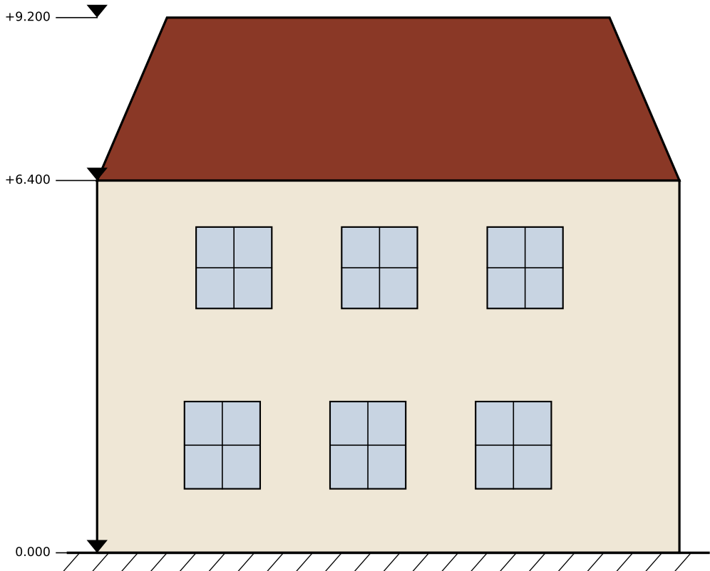
Фасад А-Г (боковой)
